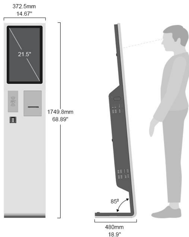
2. Rysunek wymiarowy urządzenia
